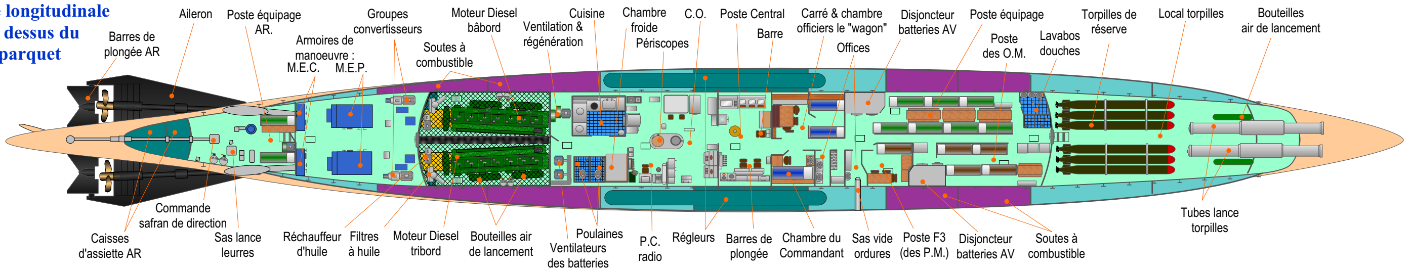
Coupe longitudinale au dessous du parquet
